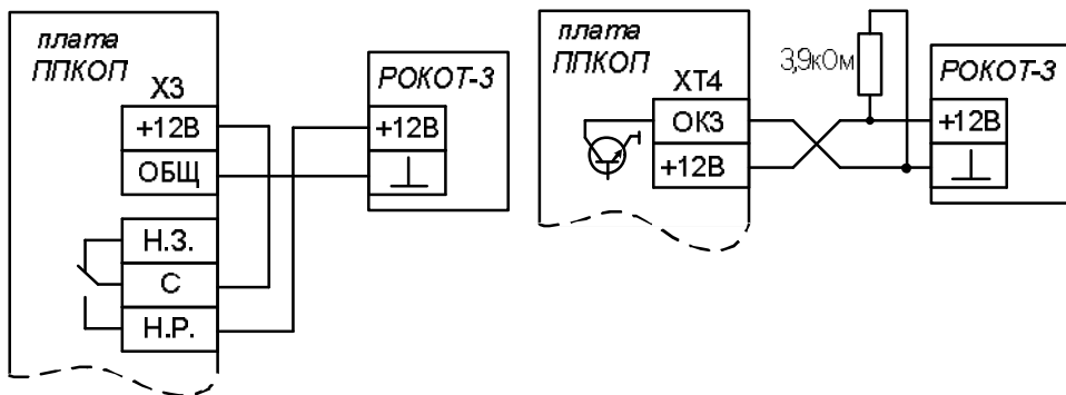
Рис. 3 Схема подключения к прибору «Циркон»
