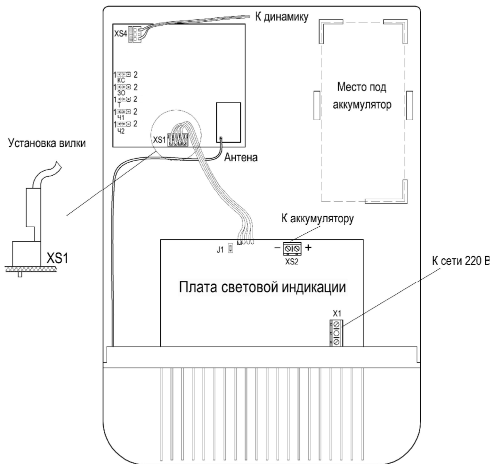
Рис. 5 Внешний вид «АС-Р2-220», крышка с динамиком снята
