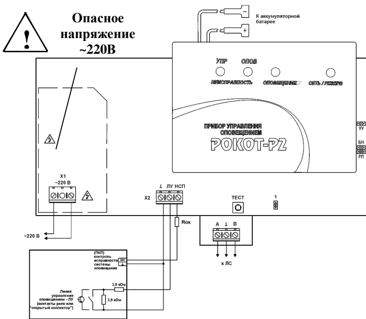
Рис. 2 Внешний вид и схема подключения ПУО «Рокот-Р2»
