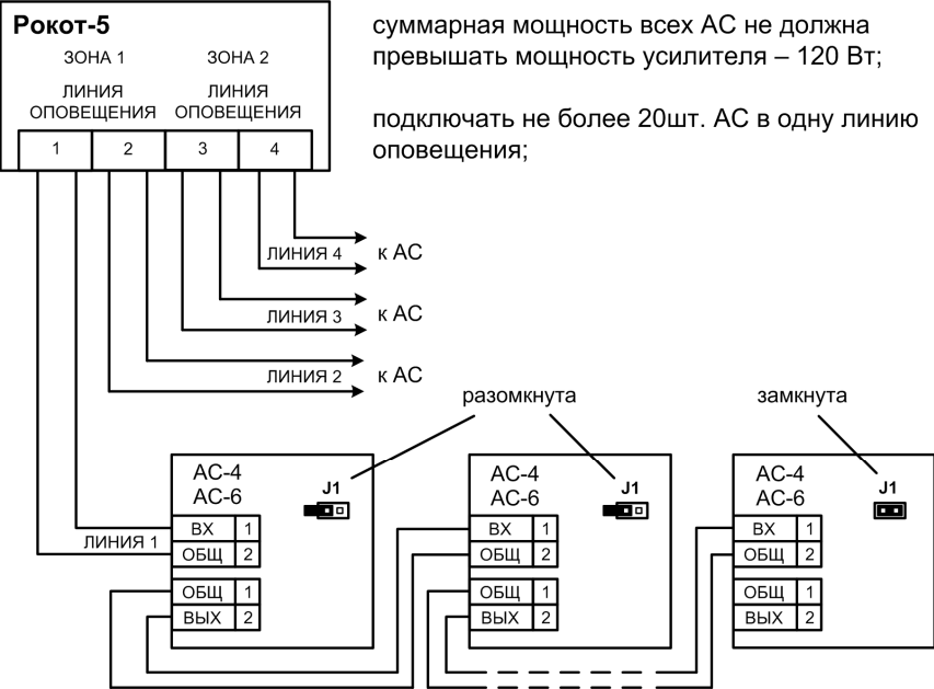
Рис.4а Схема подключений AC-4, AC-6 к линиям оповещения
