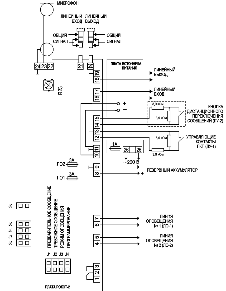
Рис. 2 Схема подключения «РОКОТ-2»
