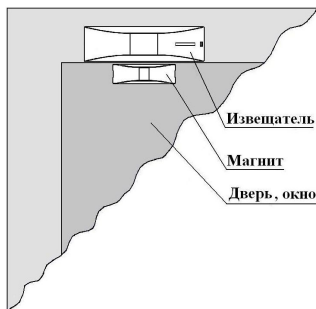
Рисунок 3.9 – Размещение на двери без металлических конструкций
