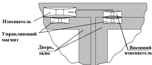
Рисунок 3.11 – Размещение на двухстворчатой двери
