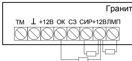
Рисунок 3.2 – Схема подключения резисторов
