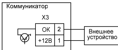
Рисунок 11.2 – Схема подключения внешнего устройства к коммуникатору
