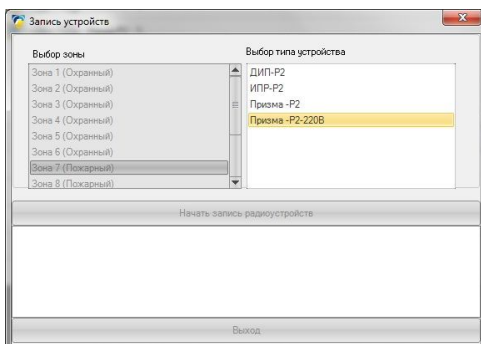
Диалоговое окно 2
