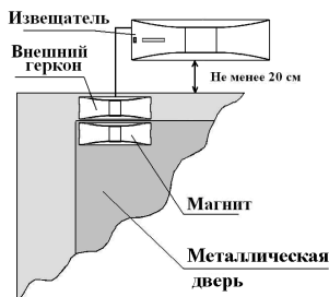
Рисунок 3.10 – Размещение на металлической двери
