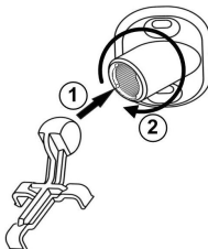
Рисунок 3.7 – Схема соединения кронштейна и держателя
