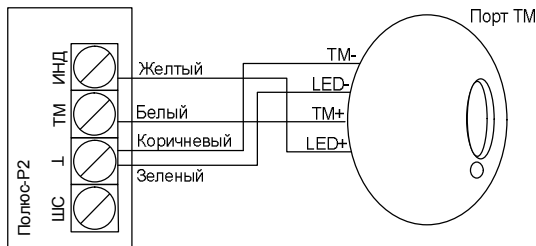
Рисунок 3.8 – Схемы подключений
