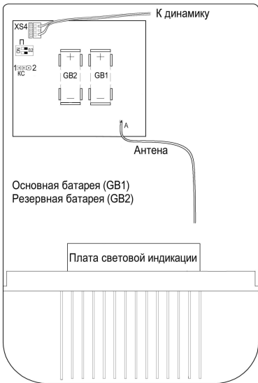
Рисунок 3.12 – Внешний вид оповещателя «Призма-Р2» (крышка с динамиком снята)
