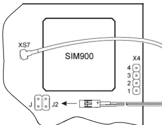
Рисунок 11.3 – Подключение термодатчика
