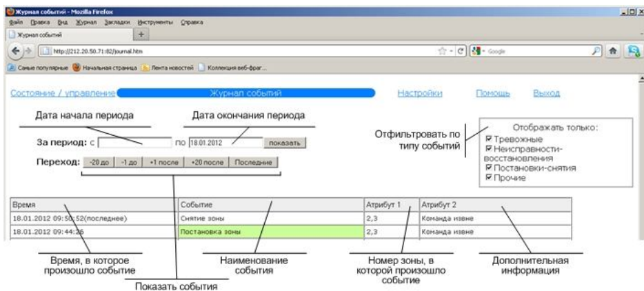
Рисунок 12.8 – Журнал событий
