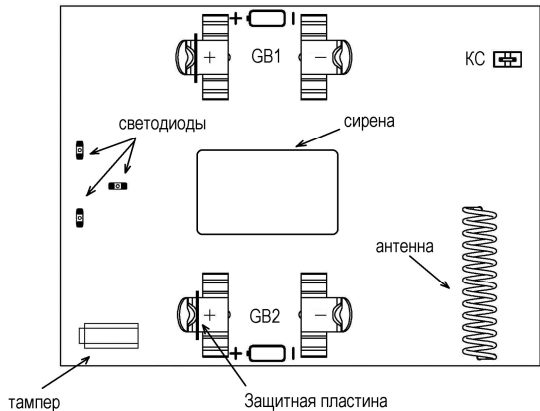
Рисунок 3.13 – Плата «Призма-P2М»
