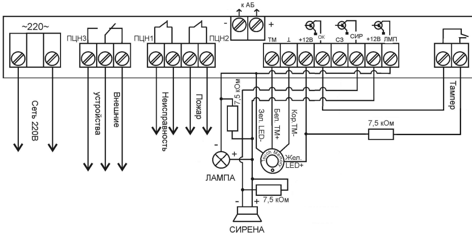
Рисунок 3.1 – Схема внешних подключений прибора
