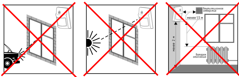
Рисунок 3.6 – Примеры неправильной установки
