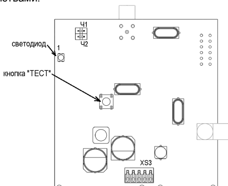
Рисунок 3.3 – Плата радиорасширителя
