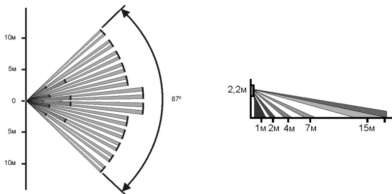
Рисунок 3.5 – Диаграмма зоны обнаружения
