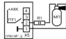
Рис 4а. Подключение модуля автоматического пожаротушения
