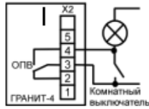
Рис 7. Подключение подсветки (1-й вариант)
