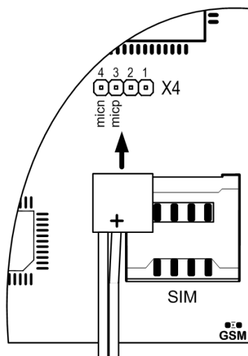
Рис.17а Подключение микрофона к коммуникатору
