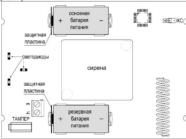
Рис.12 Плата «Призма-Р2М»
